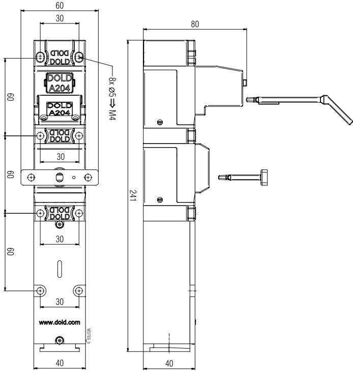
SXB01M Tolérances générales ± 2%
