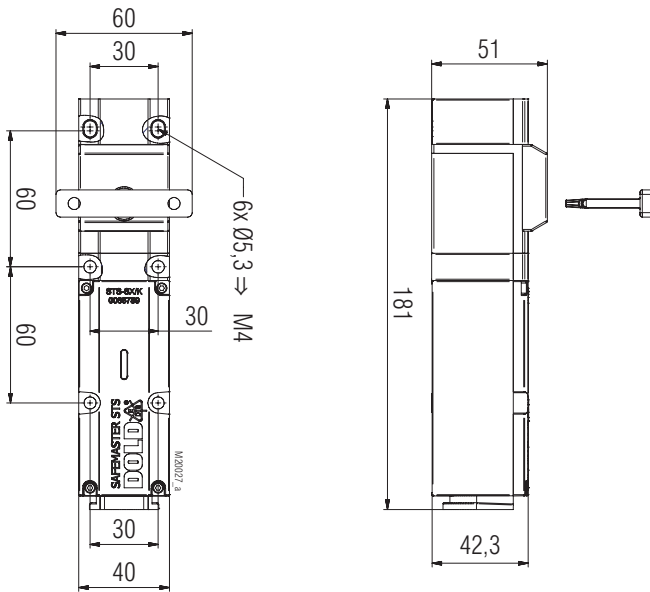
SXBM/K Tolérances générales \pm 2\%
