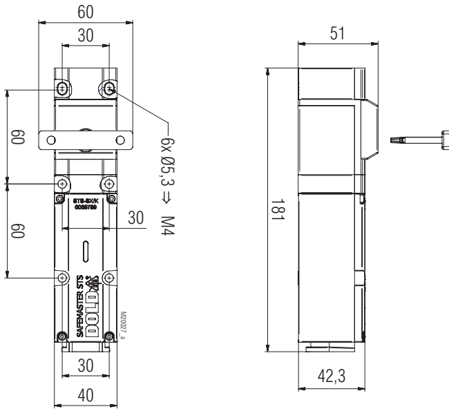
SXBM/K Freimaßtoleranzen \pm 2\%
